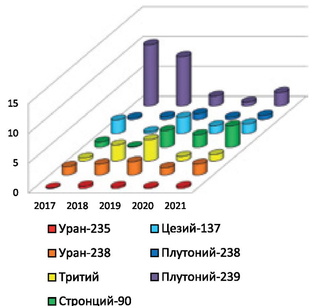
Диаграмма 3. Фактический сброс радиоактивных веществ в водные объекты в % от разрешенного сброса за 2017–2021 гг.
