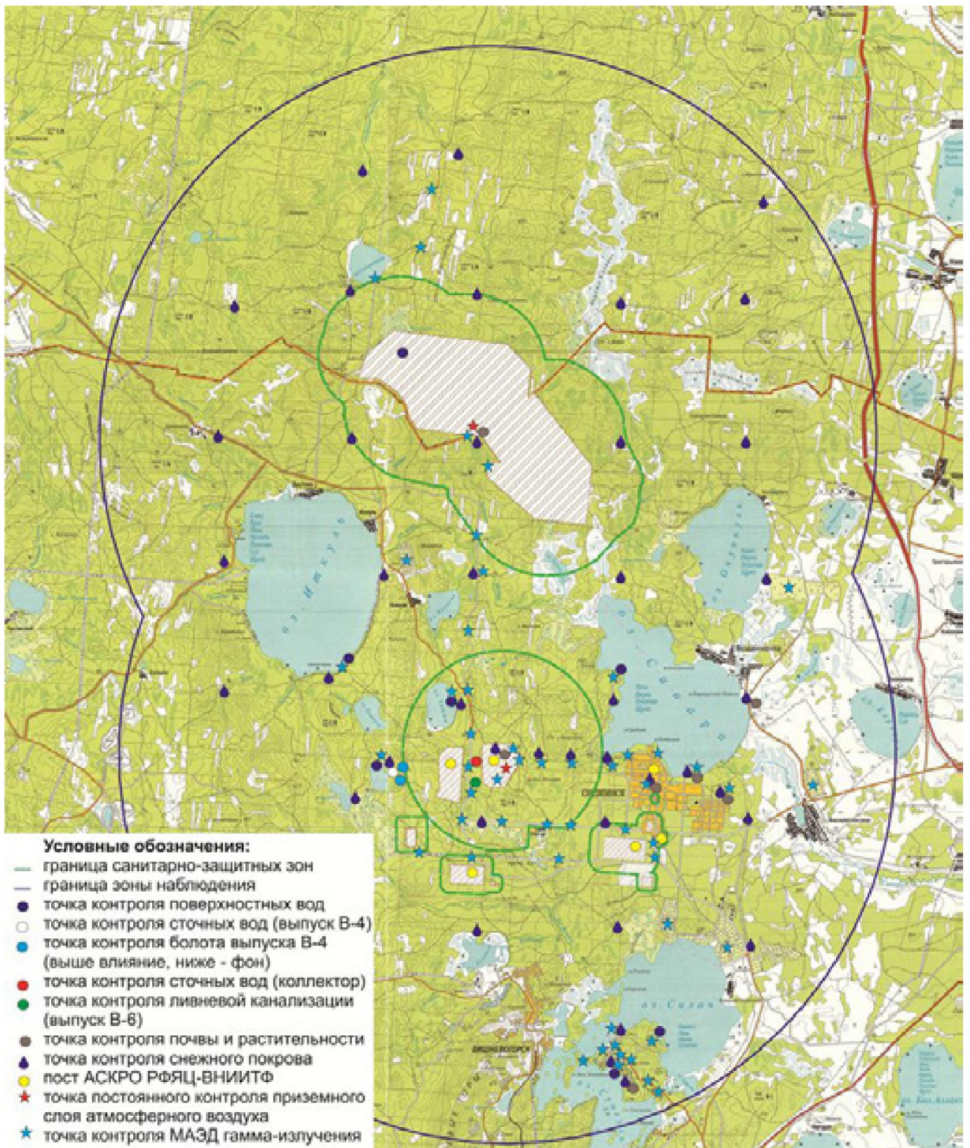
Карта-схема расположения пунктов радиационно-экологического контроля в санитарно-защитных зонах и зоне наблюдения предприятия
